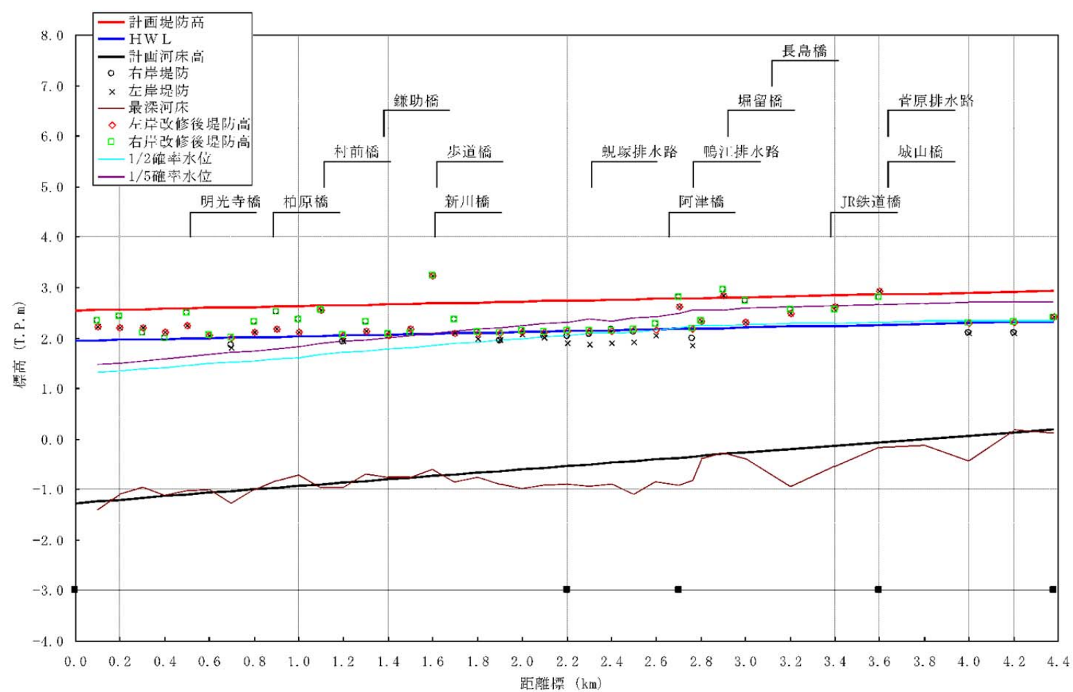
堀留川計画縦断面図
